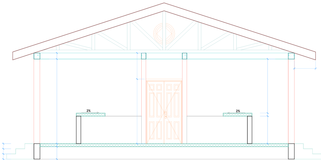
COUPE B-B
